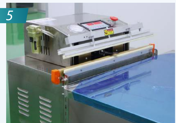
Máy hút chân không Model: VS-600
