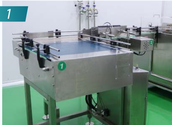
Máy cấp chai dạng băng tải Model: SSP
